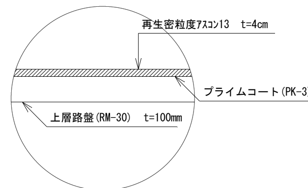
構成図 S=1:20
