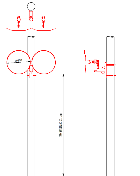
市道学校前線 S=1/50 道路反射鏡設置（電柱添加） N=1基（φ 600, 2面鏡）
