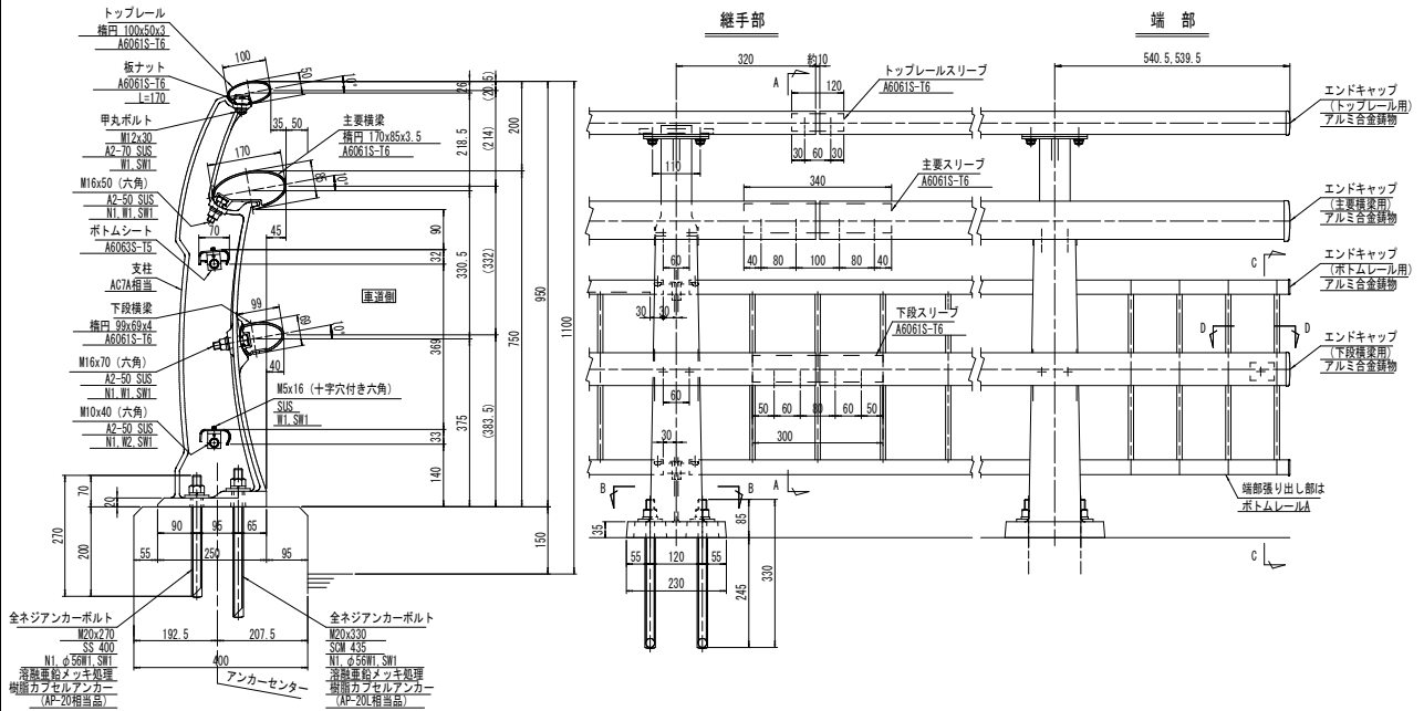
断面A-A
