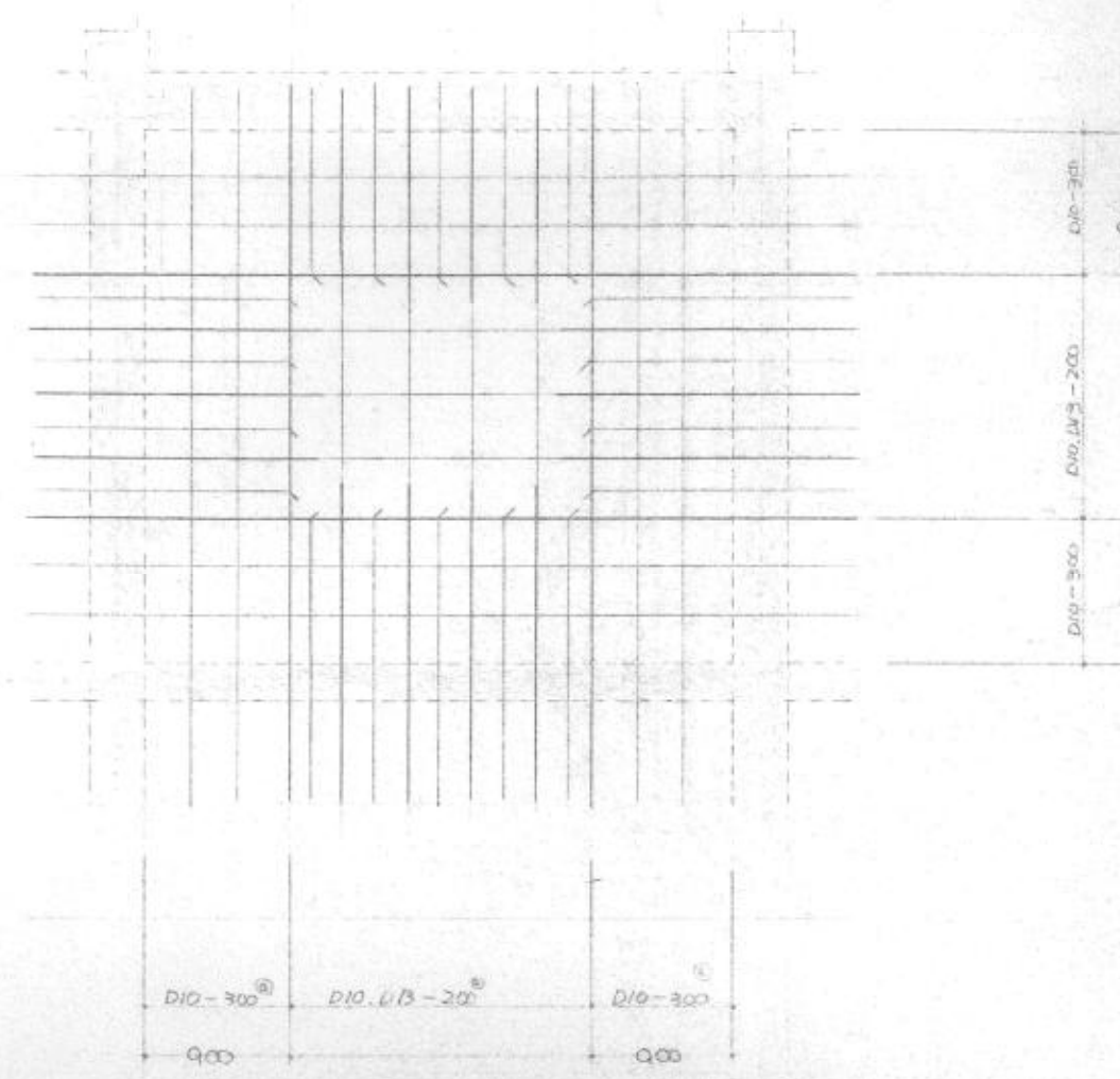
上層 ④ スラブ配筋図 1/50
