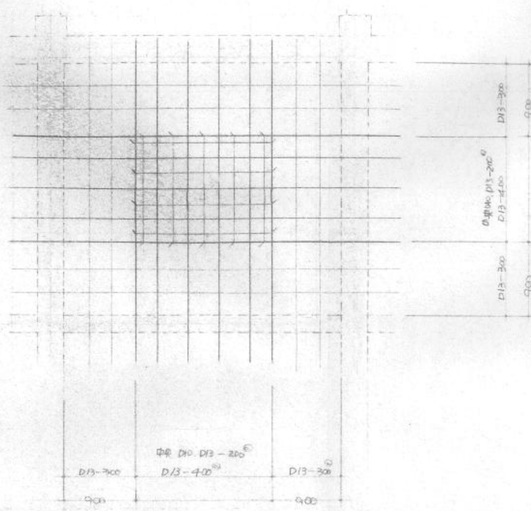
下層 ⑤ スラブ配筋図 1/50
