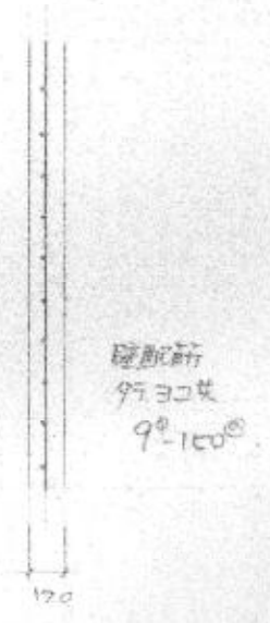
⑧ 柱配筋図 1/30
