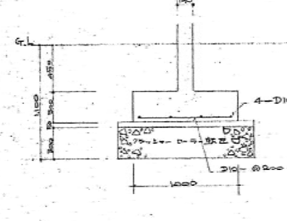
Fig. 基礎配筋図
