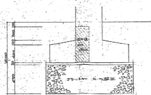
五、基礎配筋圖
