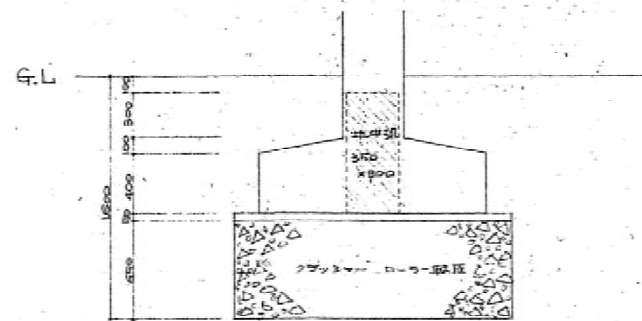
F 0 基礎配筋圖
