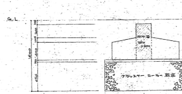
第 2 章 基礎配筋図
