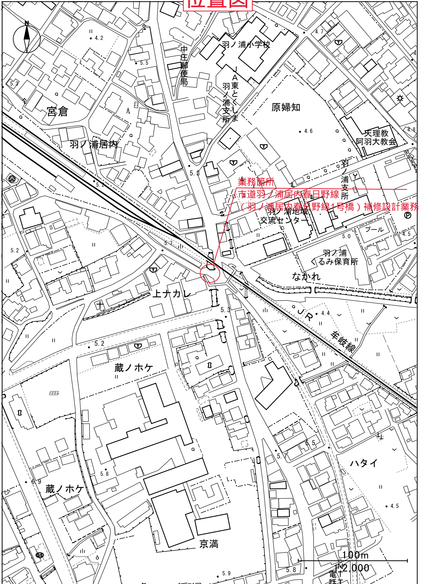
業務箇所位置図 市道羽ノ浦居内春日野線（羽ノ浦居内春日野線1号橋）補修設計業務
