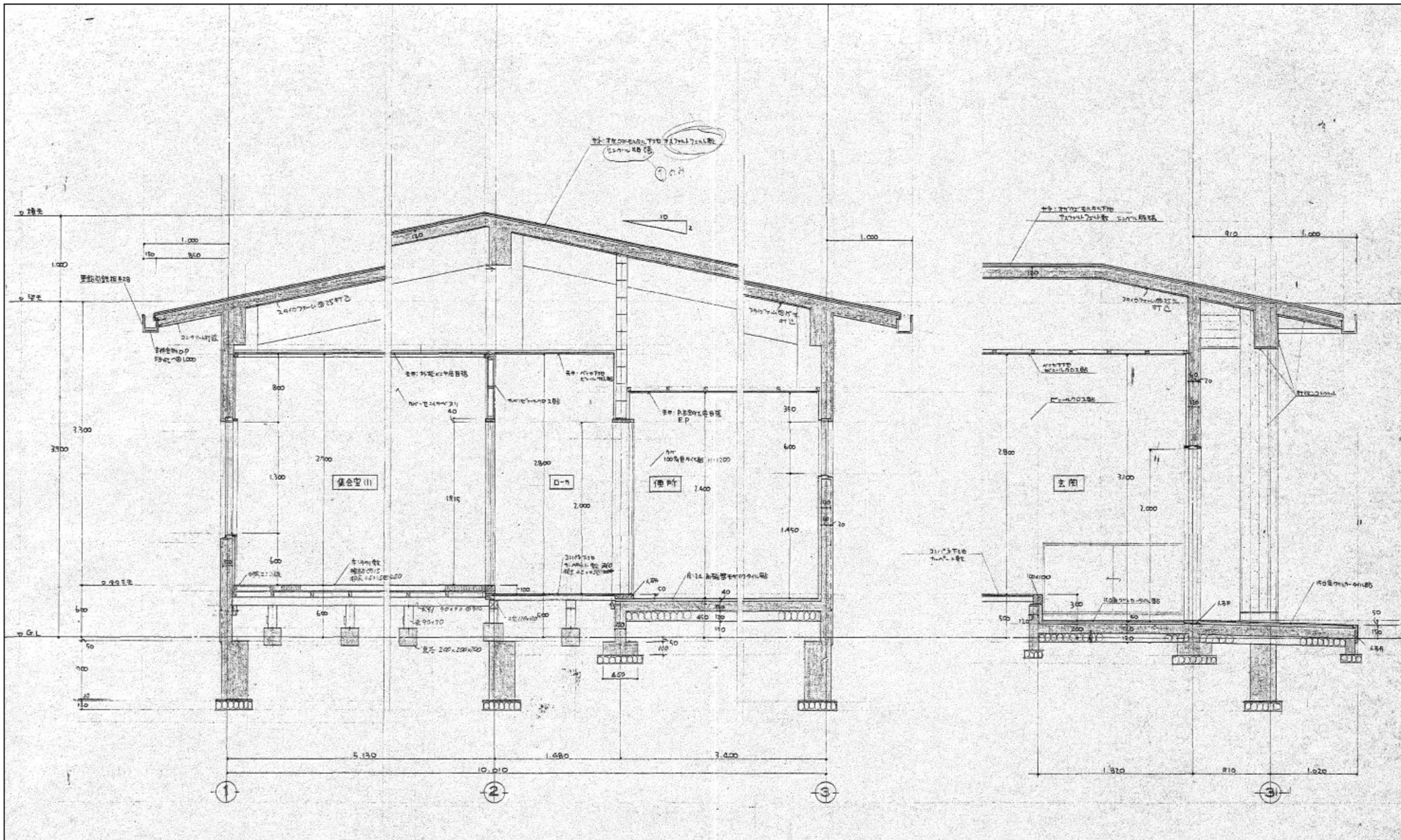
矩計図 S=1/30
