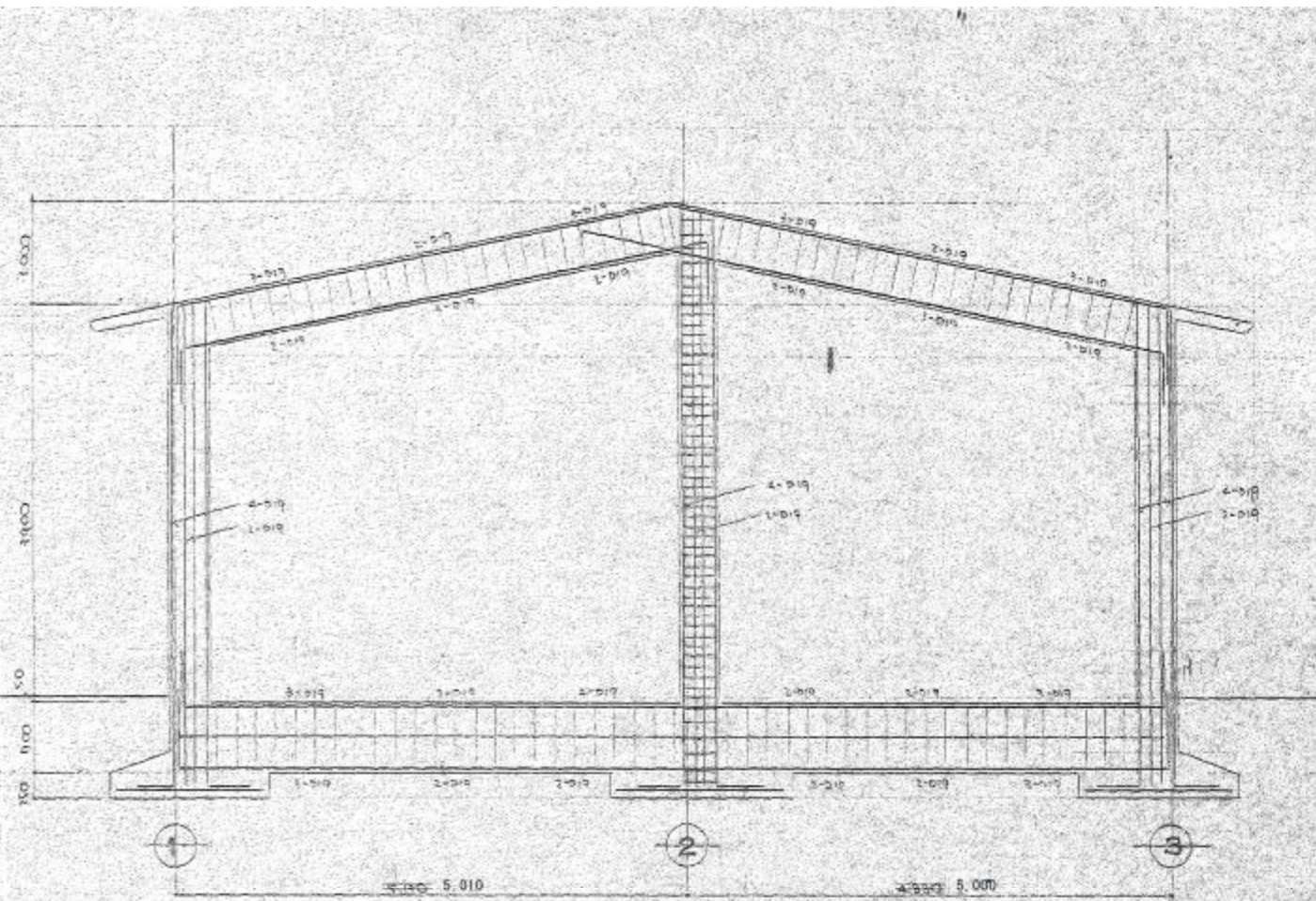
2 側面梁架配筋図
