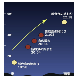
月食の行程／阿南市科学センター作図 （時刻は国立天文台暦計算室より）
