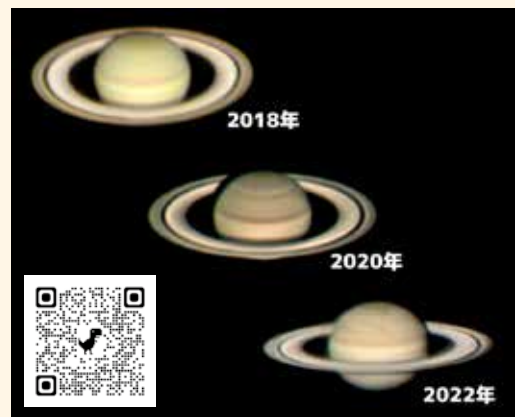
科学センターで撮影した土星の姿
