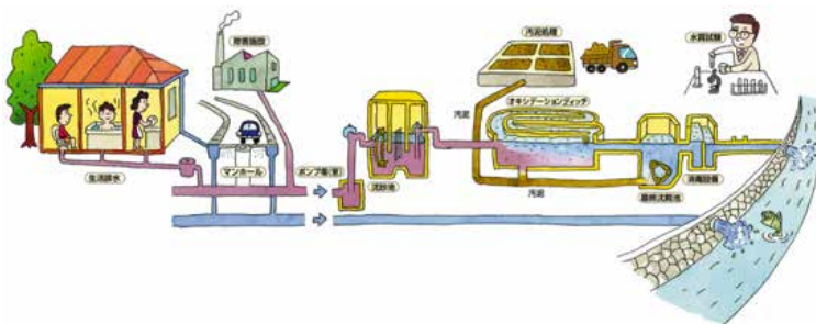
下水処理のしくみ(分流式)
