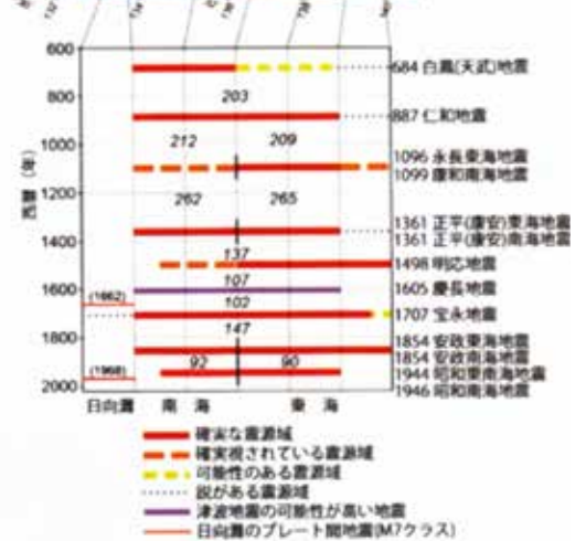
南海トラフで過去に起きた大地震の震源域の時空間分布（石橋、2002をもとに編集） ・白鳳（天武）地震（684年）以降の地震を示している。 ・図中イタリック体で表した数字は、地震の発生間隔（年）を示す。 ・震源域は地形の境界（都井岬、足摺岬、室戸岬、潮岬、大王崎、御前崎、富士川）で東西方向に区切っている。 ・黒の線棒は、南海と東海の地震が時間差（数年以内）をおいて発生したことを示す。
