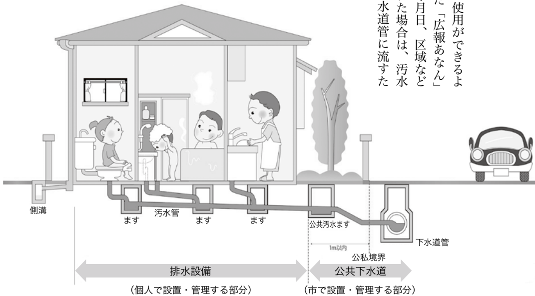
排水設備の設置例
