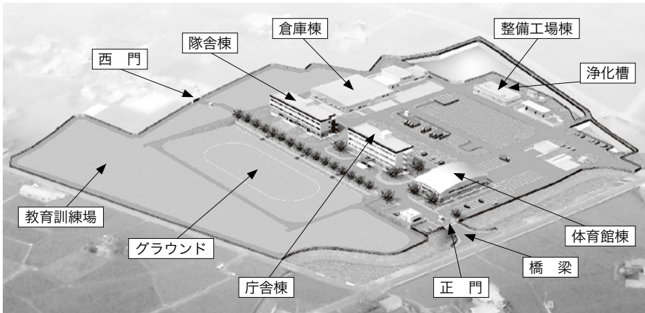
全体概略施工計画(予定)
